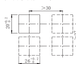
安装平装安全罩AQG16-D的开孔
