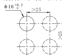
安装方形平装附件Z12的开孔
