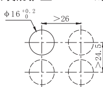
安装防护盖AQG16-B的开孔
