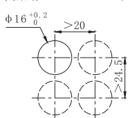
安装防护盖AQG16-A的开孔
