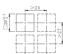
安装平装安全罩AQG16-C的开孔
