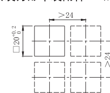
安装平装安全罩AQG16-D的开孔
