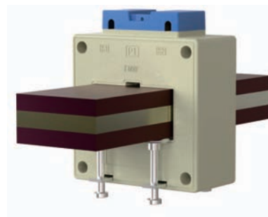
图F 双片压盘固定
