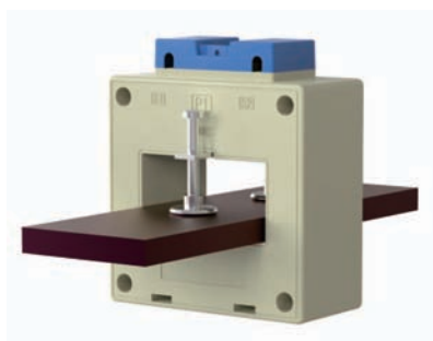
图D 单片压盘固定（直片）
